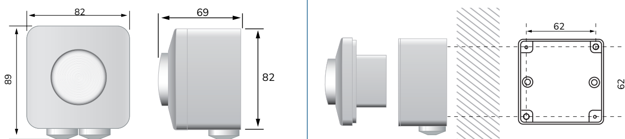
Fig. 3 Afmetingen - opbouw
