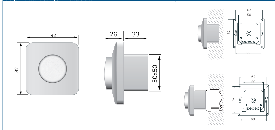
Fig. 2 Afmetingen - inbouw
